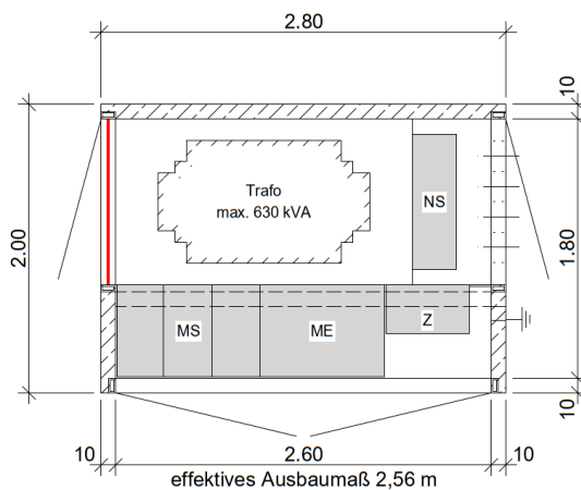
Grundriss
