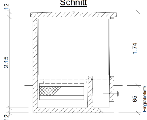
Schnitt
