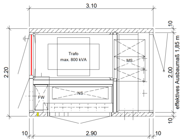
Grundriss
