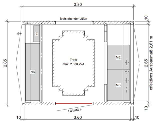
Grundriss
