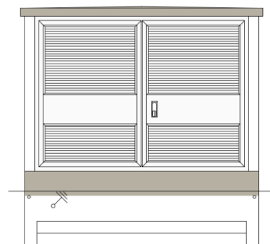
Ansicht 2
