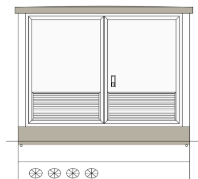
Ansicht 4
